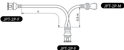
JPT-2P-M
